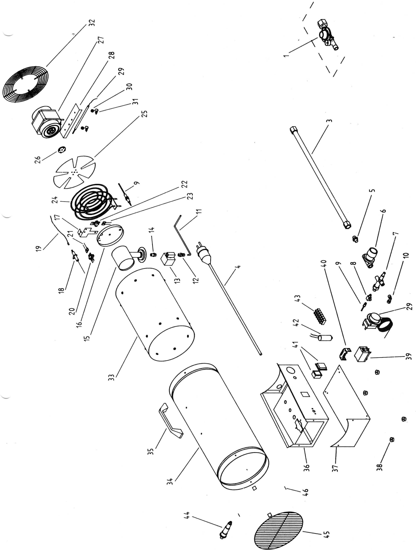
Explosionszeichnung GHE 15 M
